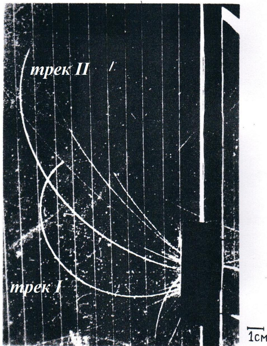
Рис. 3. Фотография треков заряженных частиц
