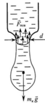
Рис. 2. Метод отрыва капль
