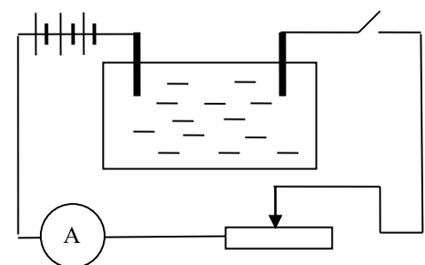
Рис. 1. Электролитическая ванна
